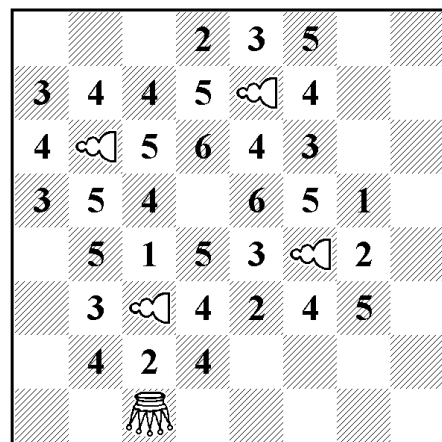
4 DU / 32 squares
