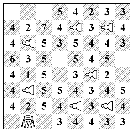
7 DU / 47 squares
